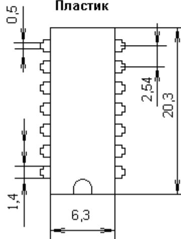
DIP14 Пластик
